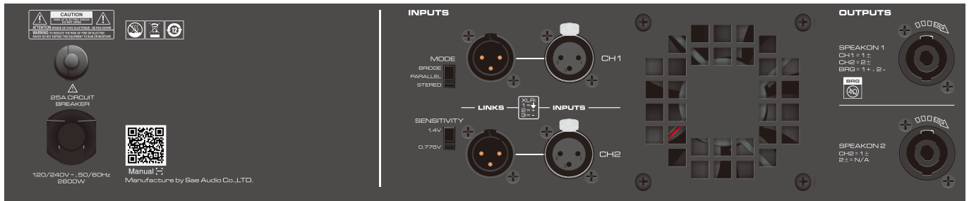
E1500 后面板
